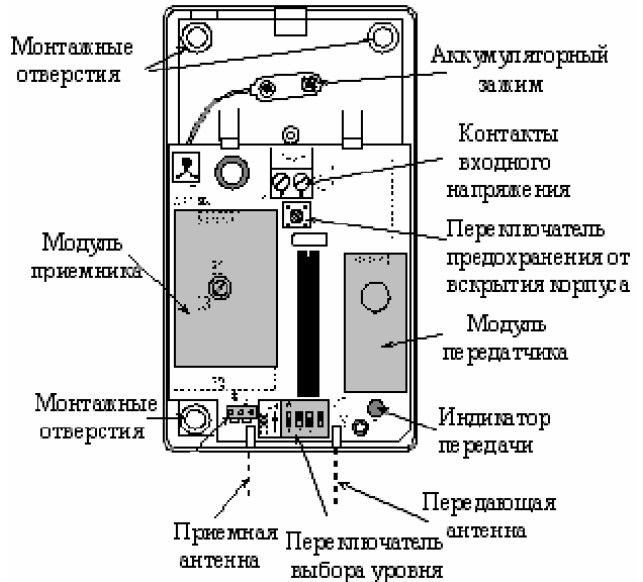
Рисунок 5. MCX-600 со снятой крышкой.
